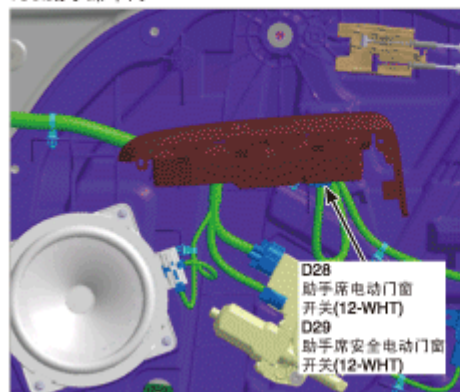
136.助手席车门
