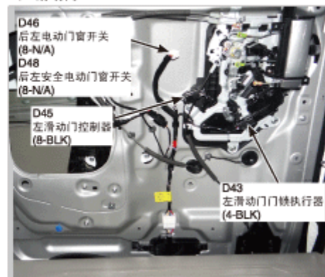
137.滑动门
