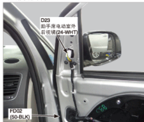
133.助手席车门
