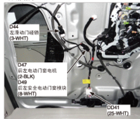
138.滑动门
